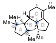
phomopsene (1)
